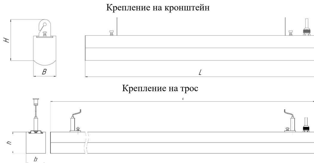
Рисунок 1 – Конструкция светильника
