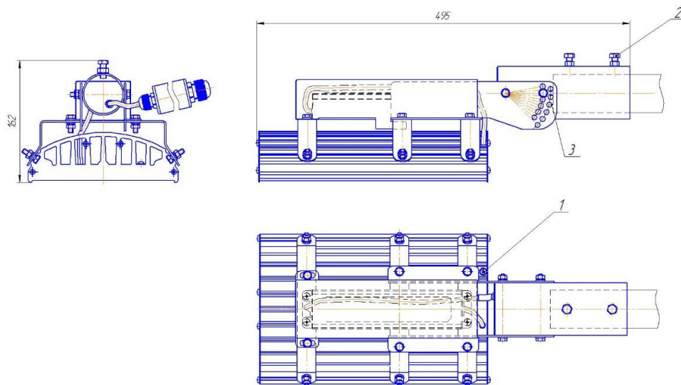
Рисунок 1 - Конструкция светильника
