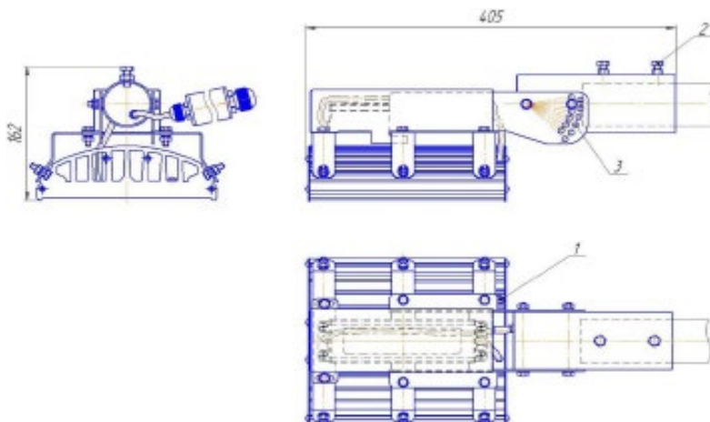
Рисунок 1 - Конструкция светильника
